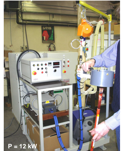
Equipement de brûlage de vernis de fils cuivre isolés
