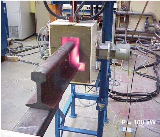
Réchauffage de rails après soudure
