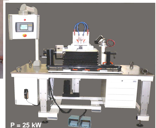
Equipement de brasage d'inserts de carbure
